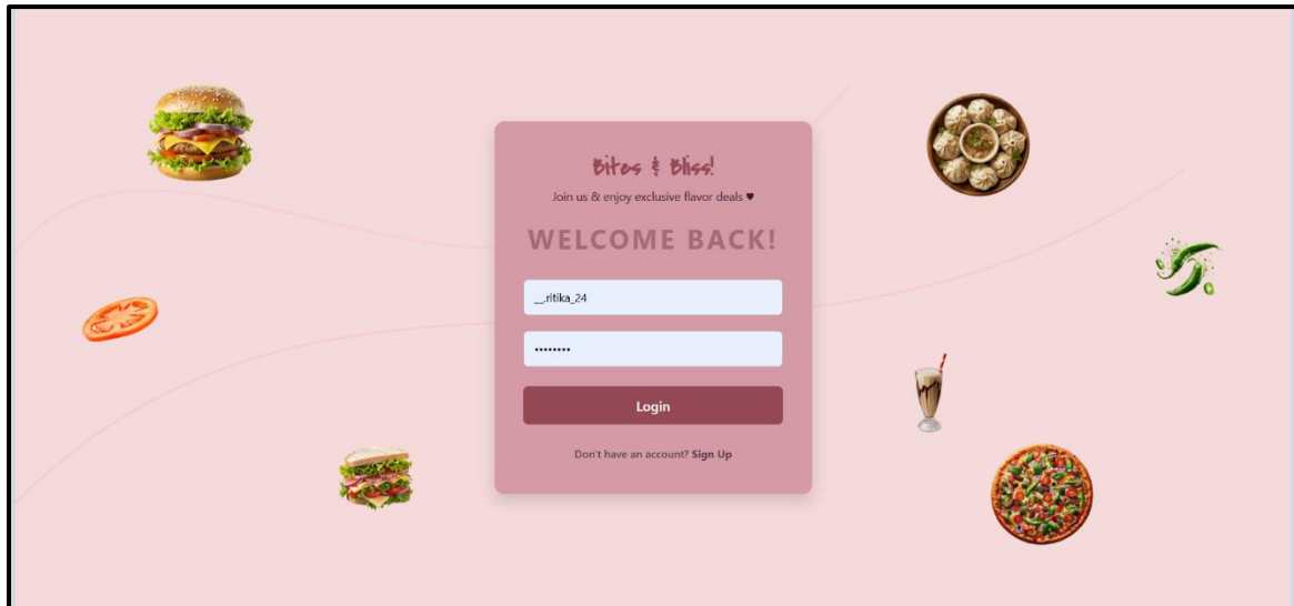
Fig. 4.7: Login Interface
